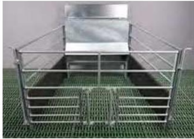
Futterautomat für Lämmer mit Schlupf
